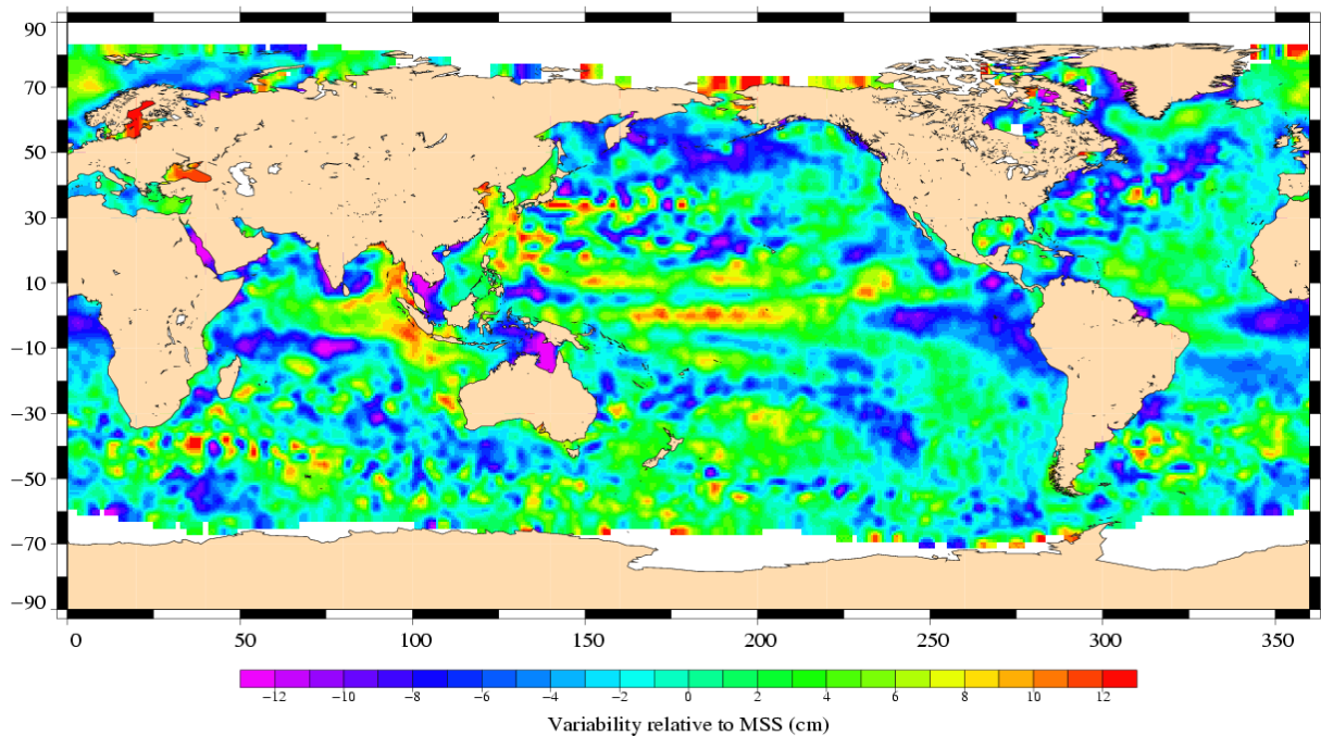
Envisat Cycle 028 21/06/2004 – 26/07/2004
