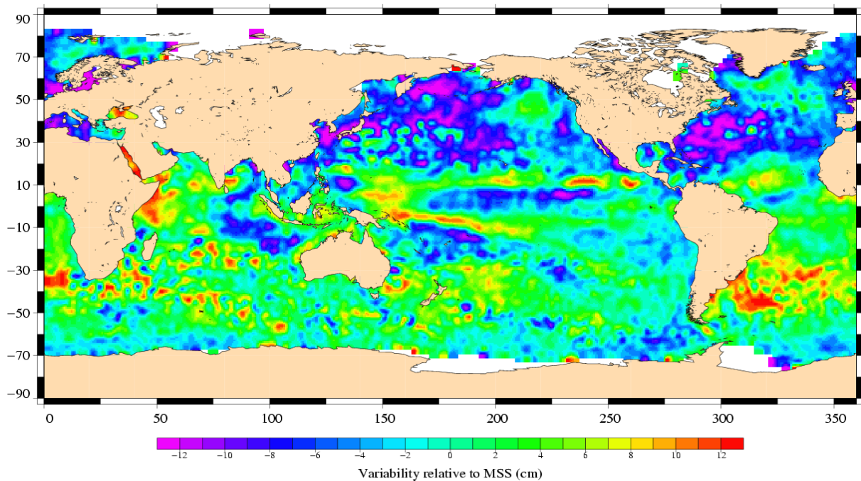
Envisat Cycle 036 28/03/2005 – 02/05/2005
