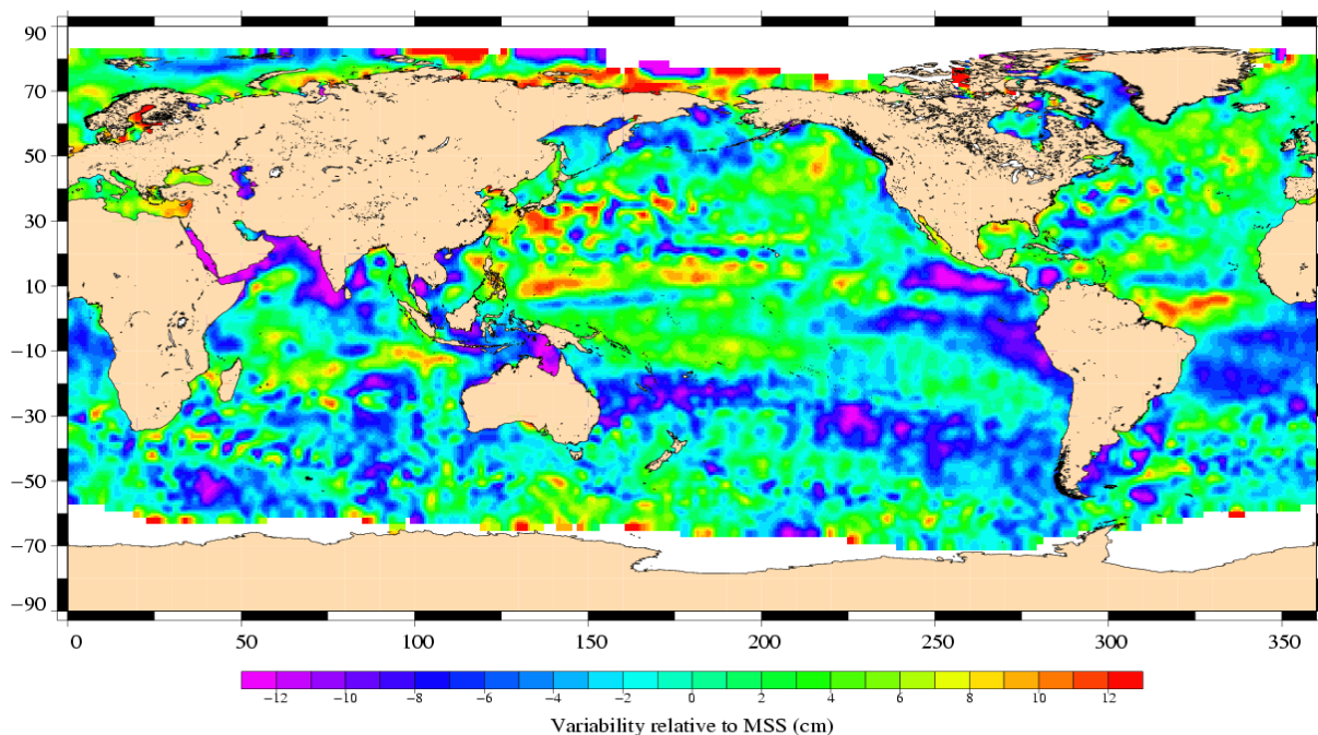
Envisat Cycle 040 15/08/2005 – 19/09/2005
