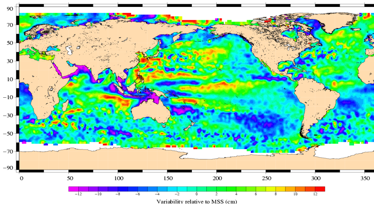
Envisat Cycle 050 31/07/2006 – 04/09/2006
