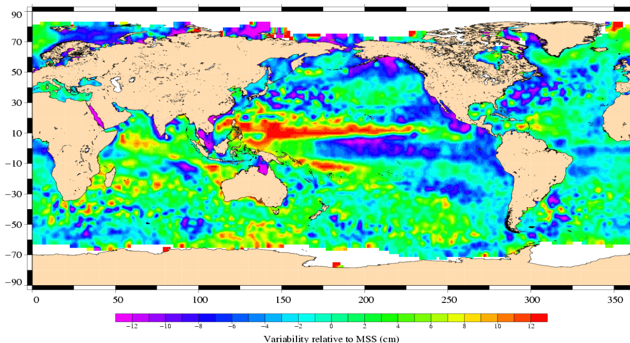
Envisat Cycle 059 11/06/2007 – 16/07/2007
