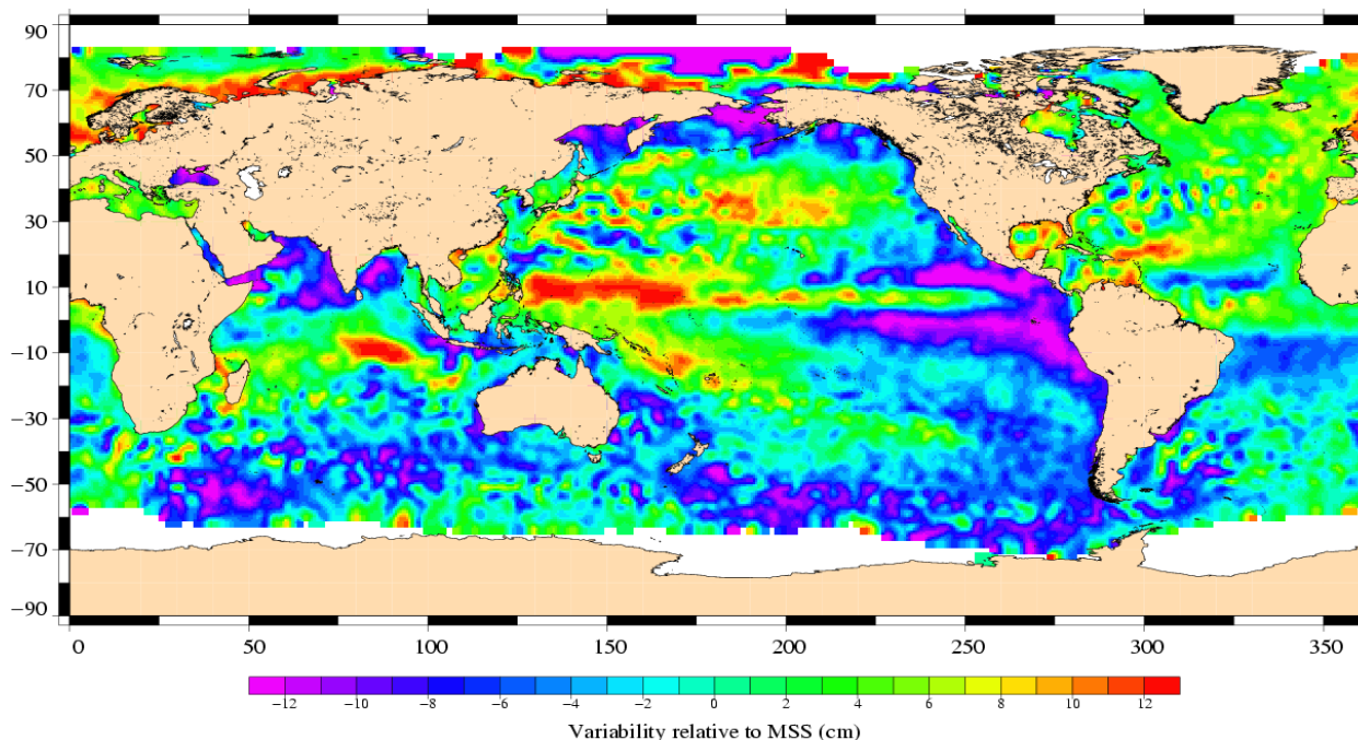
Envisat Cycle 062 27/09/2007 – 29/10/2007
