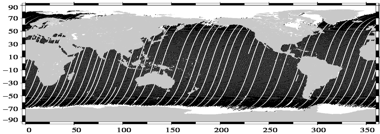
Envisat Cycle 102 (25/04/2011 / 25/05/2011)
