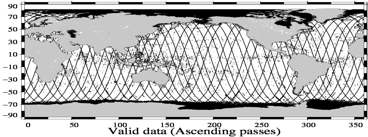
Envisat Cycle 102 (25/04/2011 / 25/05/2011)
