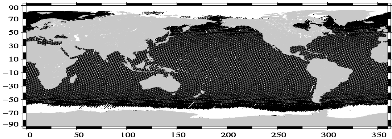
Valid data (Descending passes) Envisat Cycle 108 (22/10/2011 / 21/11/2011)
