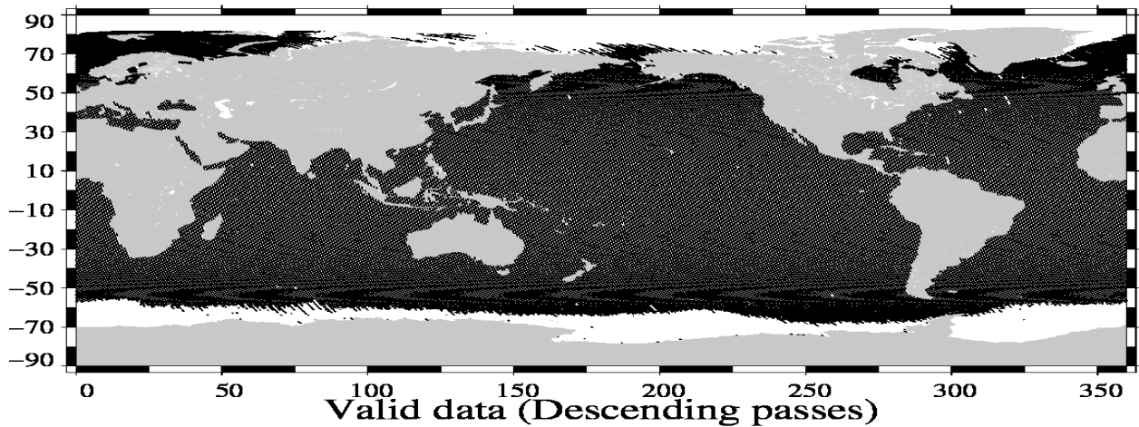
Valid data (Descending passes) Envisat Cycle 108 (22/10/2011 / 21/11/2011)
