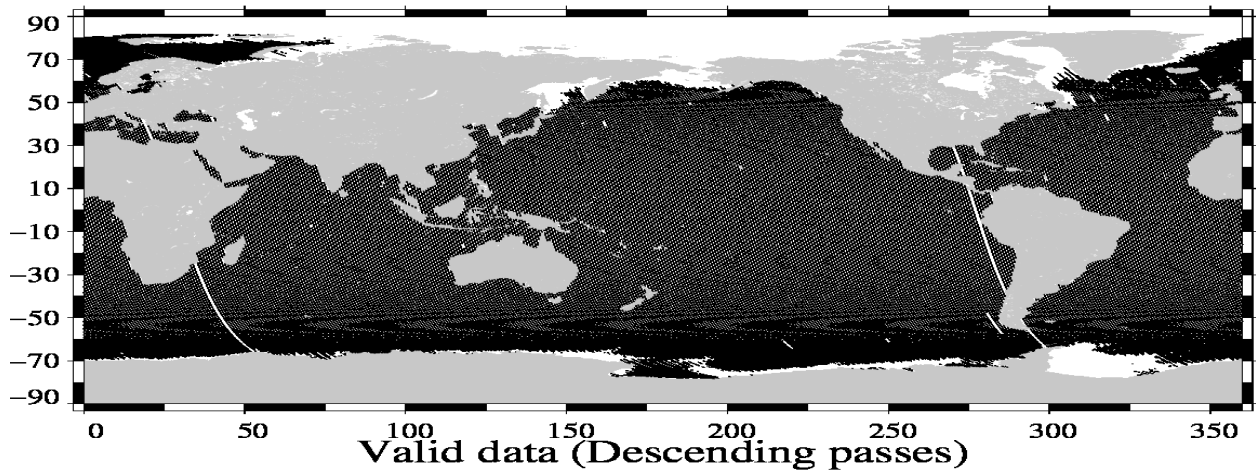
Valid data (Descending passes) Envisat Cycle 112 (19/02/2012 / 20/03/2012)
