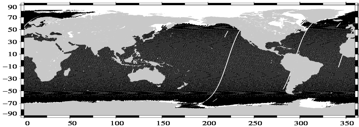
Valid data (Descending passes) Envisat Cycle 112 (19/02/2012 / 20/03/2012)
