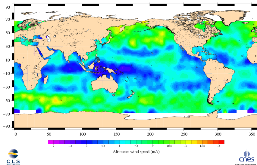
Jason-1 Cycle 143 23/11/2005 - 03/12/2005
