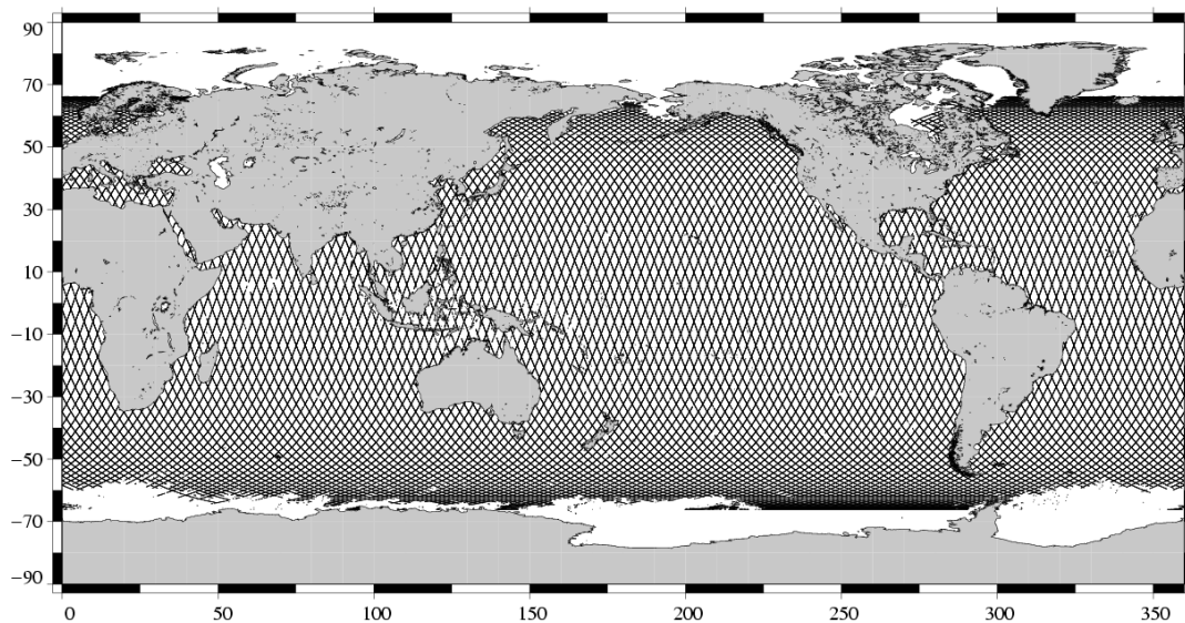
Valid data Jason-1 Cycle 144 (03/12/2005 / 13/12/2005)
