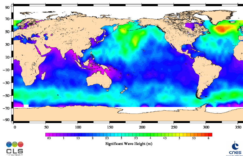
Jason-1 Cycle 255 07/12/2008 - 17/12/2008
