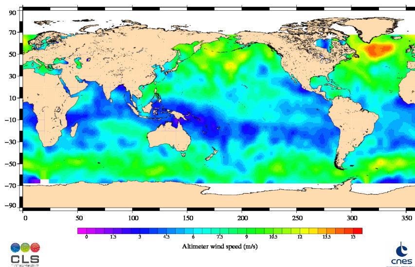
Jason-1 Cycle 255 07/12/2008 - 17/12/2008
