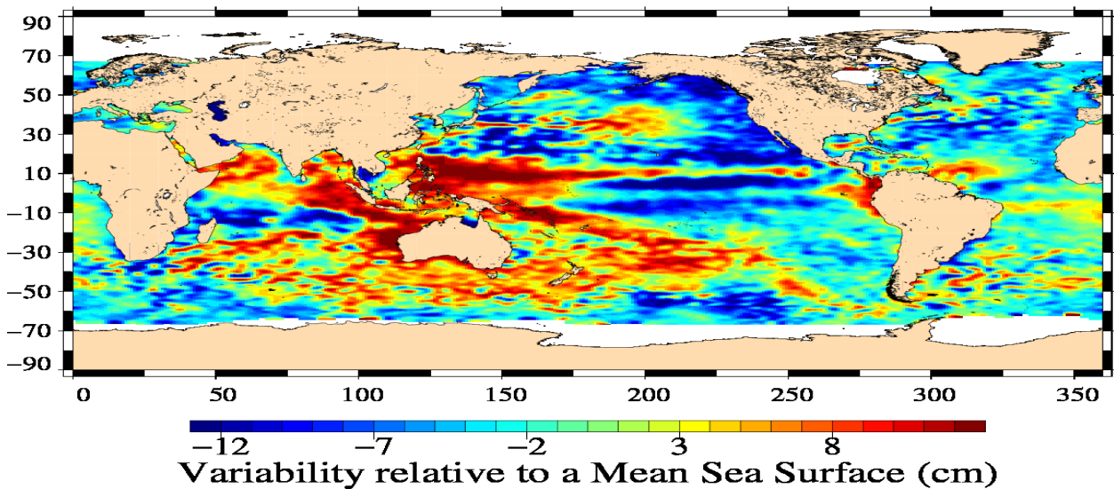
Jason-1 Cycle 501 18/05/2012 – 29/05/2012
