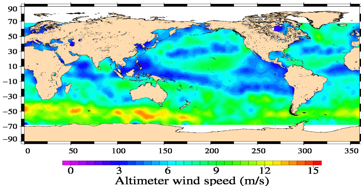
Jason-1 Cycle 501 18/05/2012 – 29/05/2012
