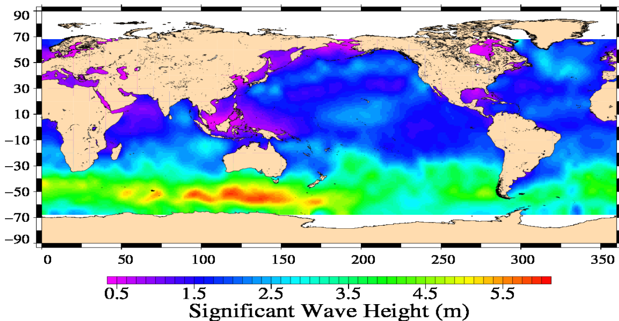
Jason-1 Cycle 501 18/05/2012 – 29/05/2012
