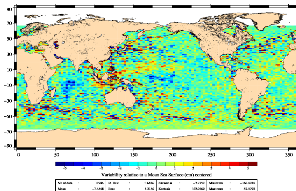
Jason-1 – Jason-2 (Cycle 022 to 094)
