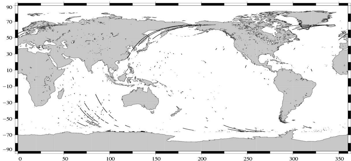
Edited parameter : Radiometer wet tropospheric correction T/P Cycle 408 (11/10/2003 / 21/10/2003)
