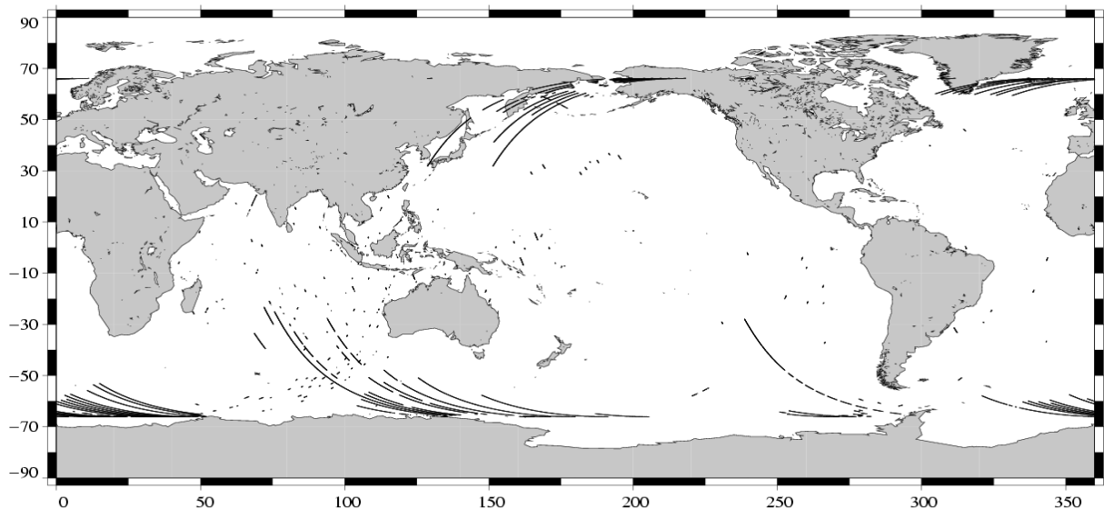
Edited parameter : Radiometer wet tropospheric correction T/P Cycle 423 (08/03/2004 / 18/03/2004)
